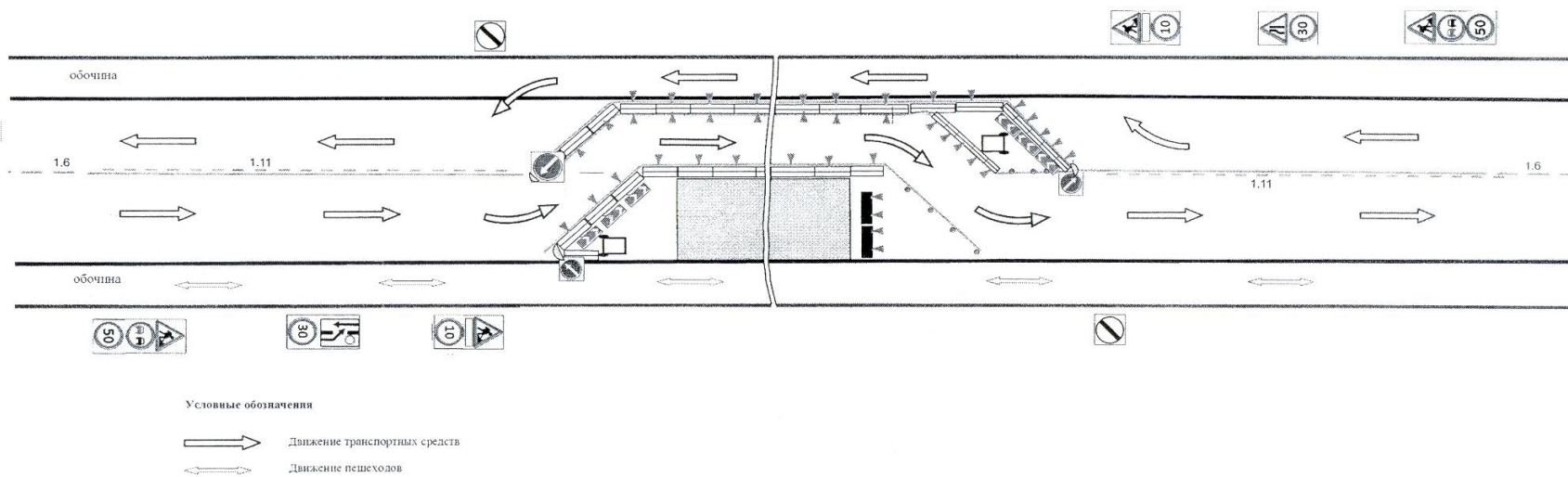
План схема движения транспортных средств и людей при проведении дорожно-строительных работ
